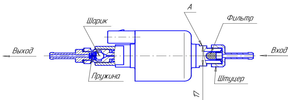
Рис. 5 – Топливный насос
